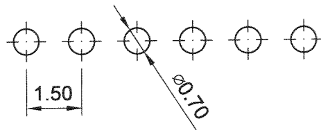
P.C.Board Layout
